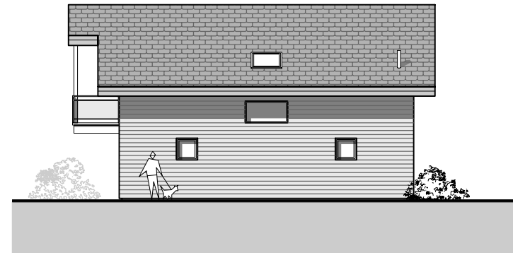
Façade Est
