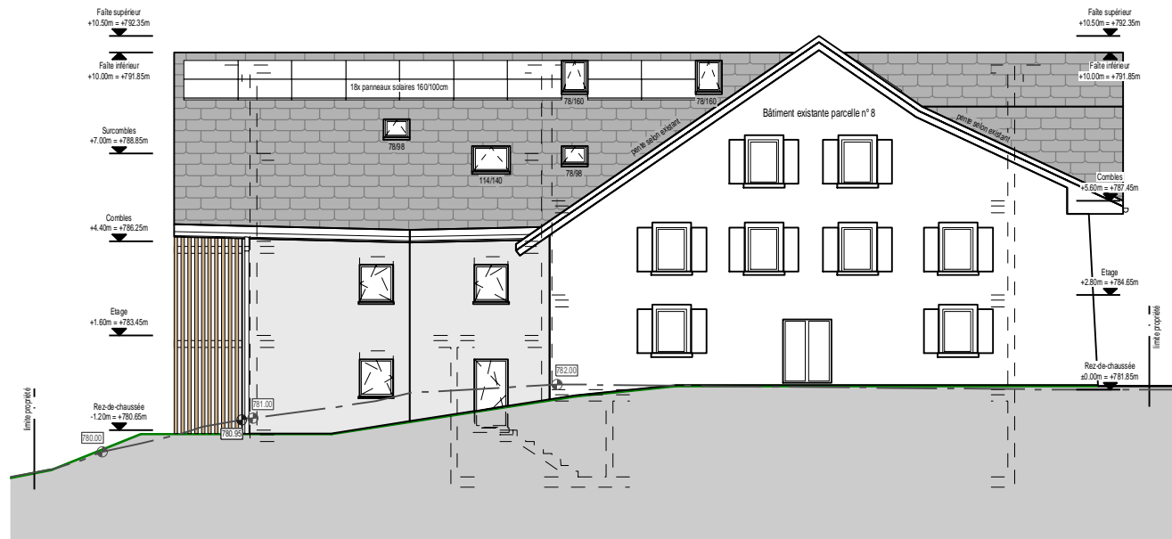
Façade Ouest
