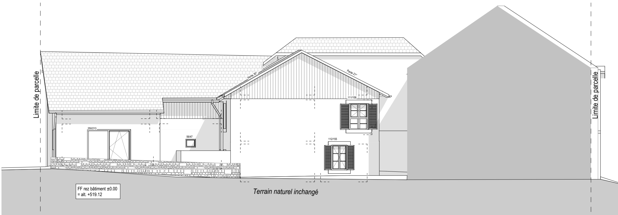
Façade est
