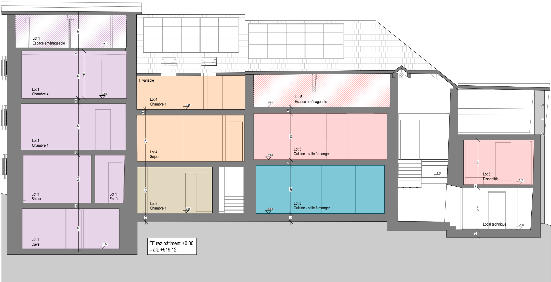
Coupe AA
