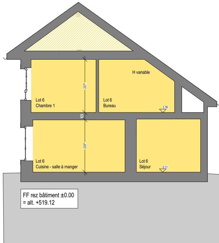
Coupe BB
