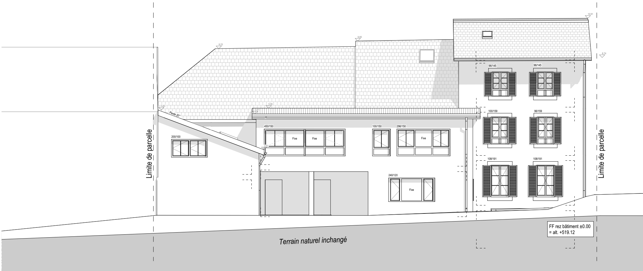
Façade nord
