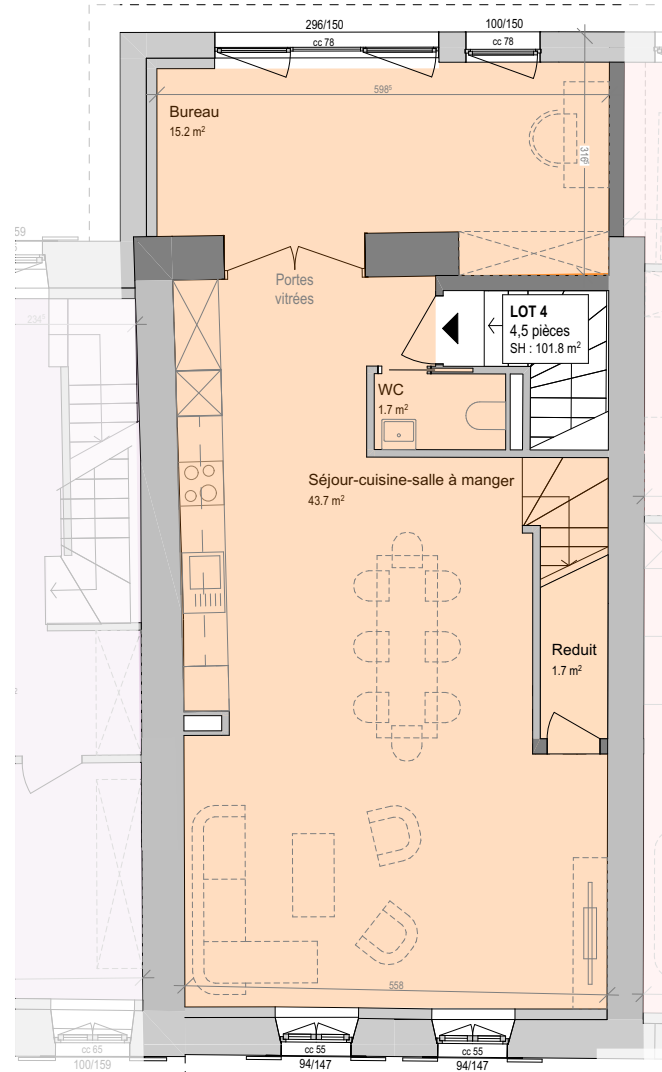
Etage 1
