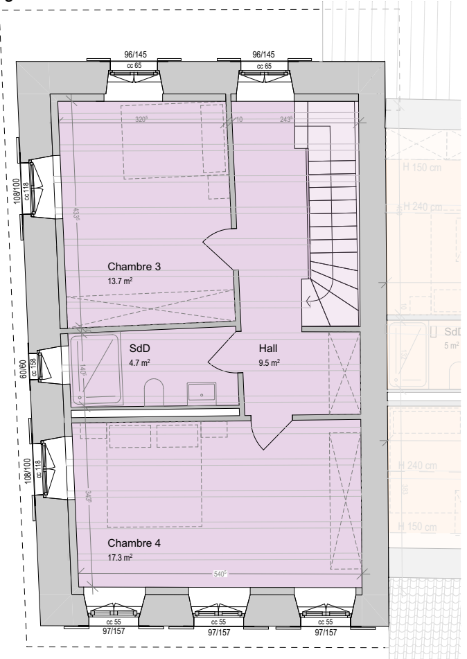
Etage 2
