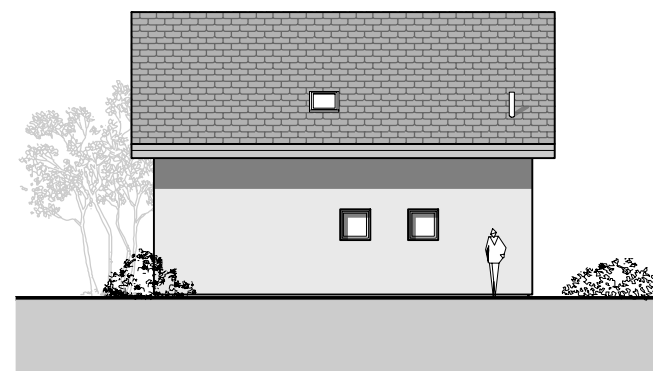
Façade Est
