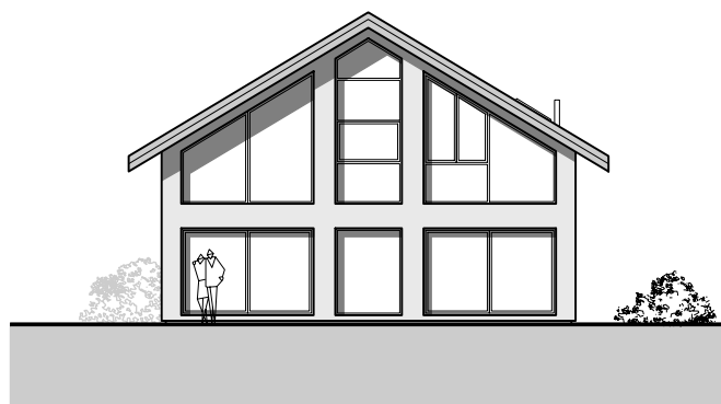
Façade Sud
