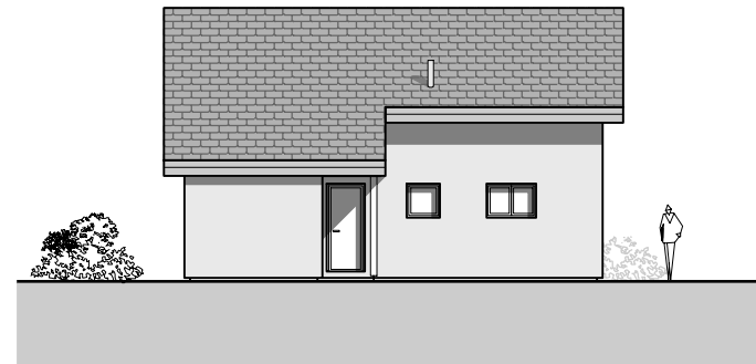
Façade Ouest
