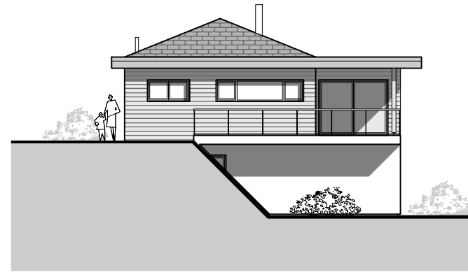
Façade Ouest
