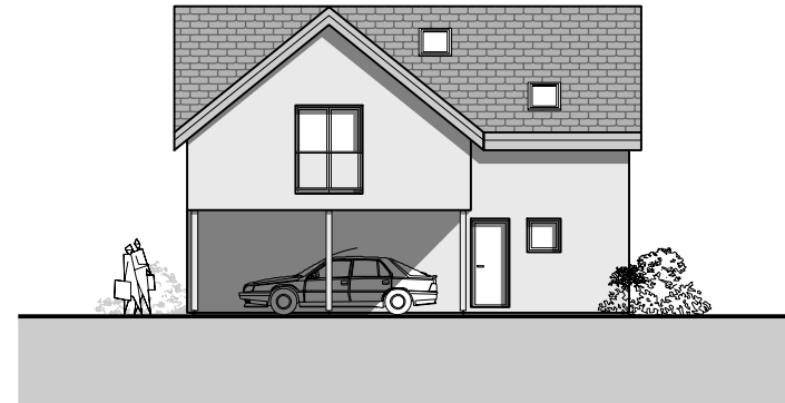
Façade Est
