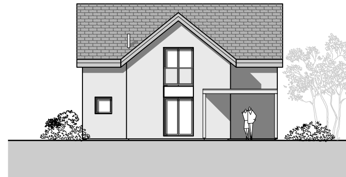
Façade Ouest
