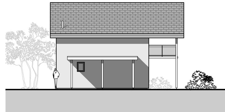
Façade Ouest
