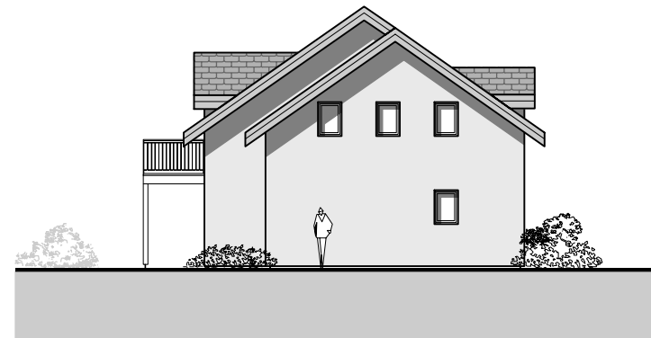
Façade Est
