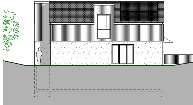
Façade Ouest
