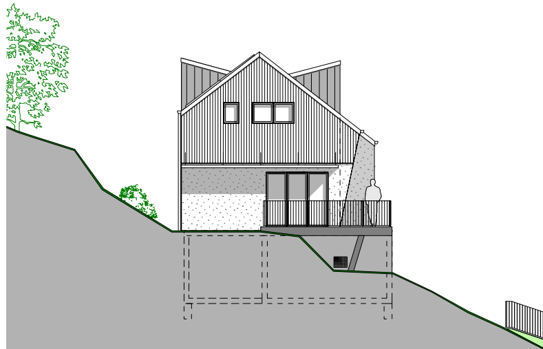
Façade Sud
